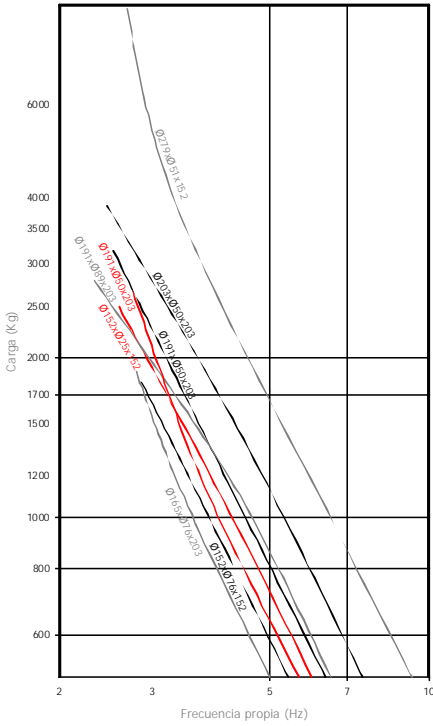
FRECUENCIA PROPIA AMC MECANOCUCHO® MUELLES ELASTOMÉRICOS REFORZADOS Ø152 - Ø279
