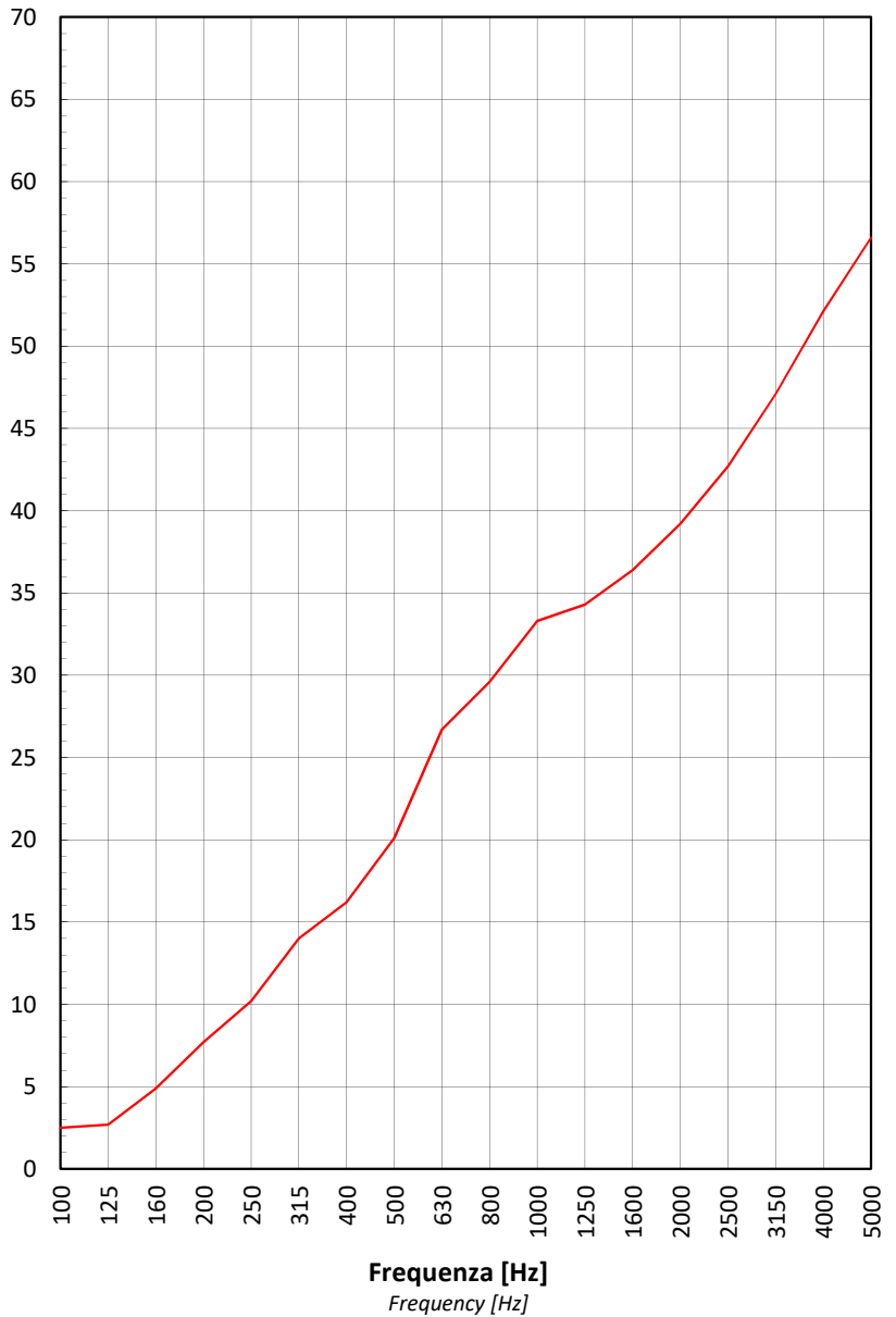
Riduzione del livello di pressione sonora di calpestio "ΔL" [dB] Reduction in impact sound pressure level "ΔL" [dB]
