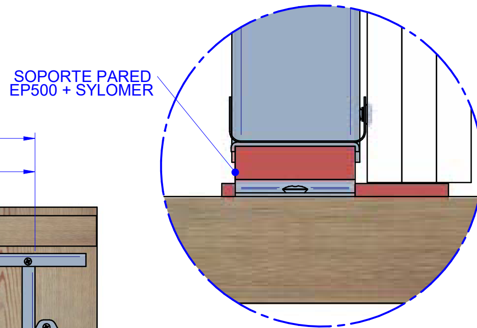
DETALLE B
