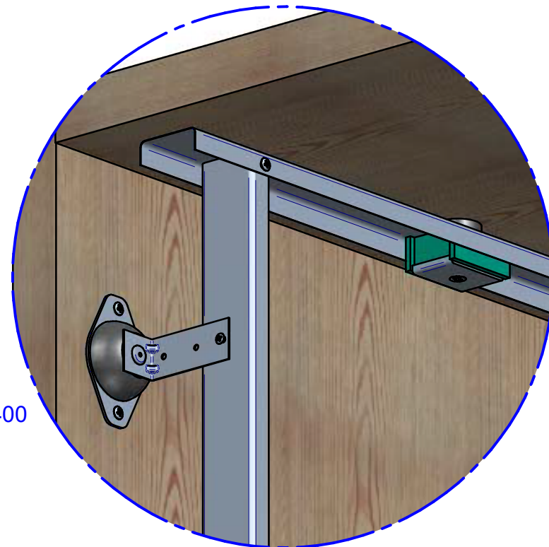
DETALLE A
