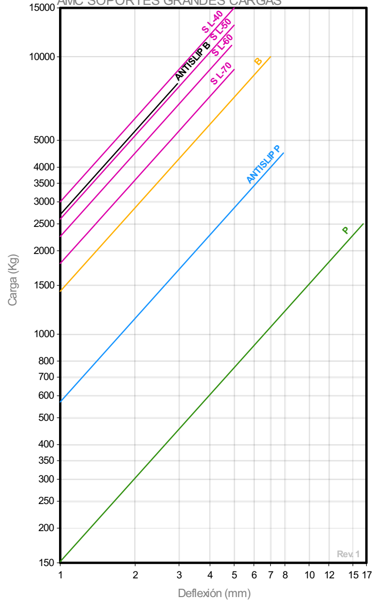
CURVAS DE CARGA FLECHA AMC SOPORTES GRANDES CARGAS
