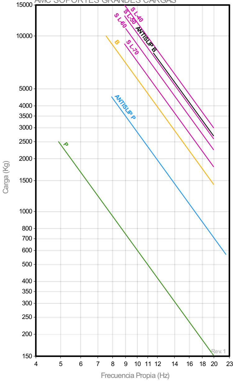
FRECUENCIA PROPIA AMC SOPORTES GRANDES CARGAS
