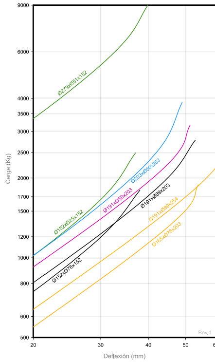
CURVAS DE CARGA FLECHA AMC MECANOCAUCHO® MUELLES ELASTOMÉRICOS REFORZADOS Ø152 - Ø279
