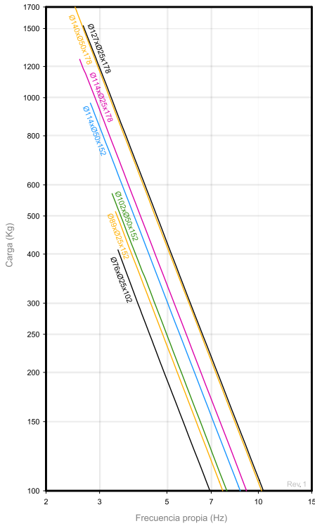
FRECUENCIA PROPIA AMC MECANOCAUCHO® MUELLES ELASTOMÉRICOS REFORZADOS Ø76 - Ø140
