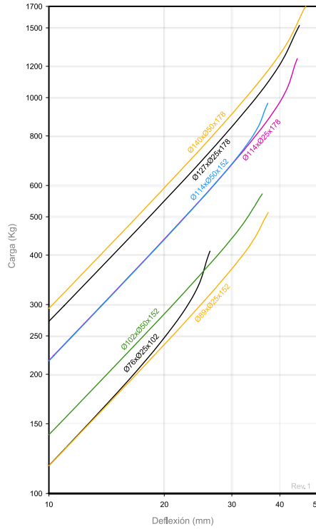
CURVAS DE CARGA FLECHA AMC MECANOCAUCHO® MUELLES ELASTOMÉRICOS REFORZADOS Ø76 - Ø140
