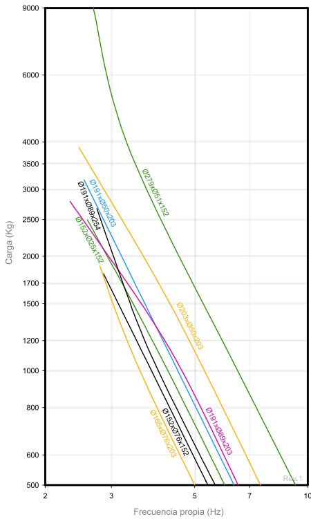
FRECUENCIA PROPIA AMC MECANOCAUCHO® MUELLES ELASTOMÉRICOS REFORZADOS Ø152 - Ø279
