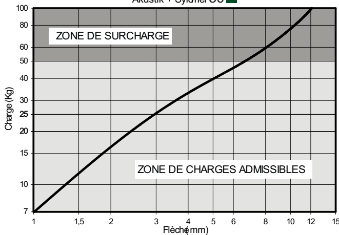
Akustik + Sylomer 50
