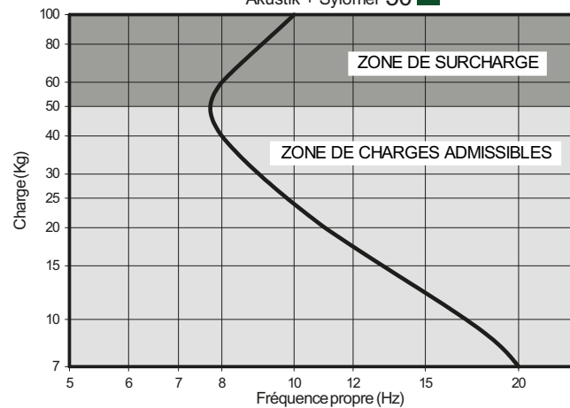
Akustik + Sylomer 50
