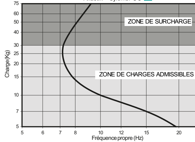
Akustik + Sylomer 50
