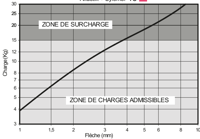
Akustik + Sylomer 30
