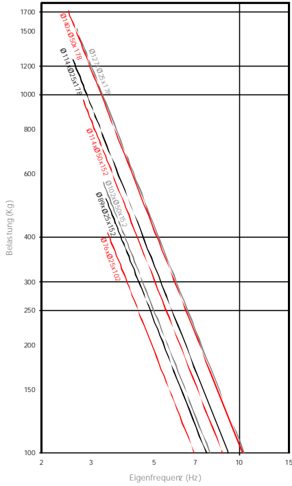
EIGENFREQUENZEN AMC MECANOCAUCHO® VERSTÄRKTE ELASTOMERFEDERN Ø76 - Ø140
