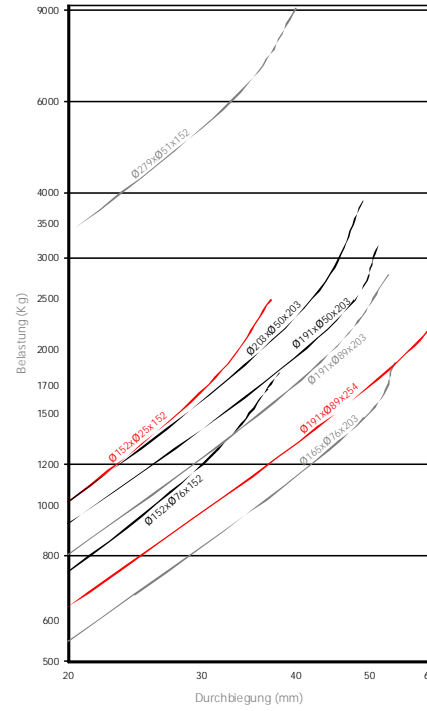
BELASTUNGSKURVEN DURCHBIEGUNG AMC MECANOCAUCHO® VERSTÄRKTE ELASTOMERFEDERN Ø152 - Ø279
