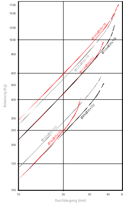
BELASTUNGSKURVEN DURCHBIEGUNG AMC MECANOCAUCHO® VERSTÄRKTE ELASTOMERFEDERN Ø76 - Ø140
