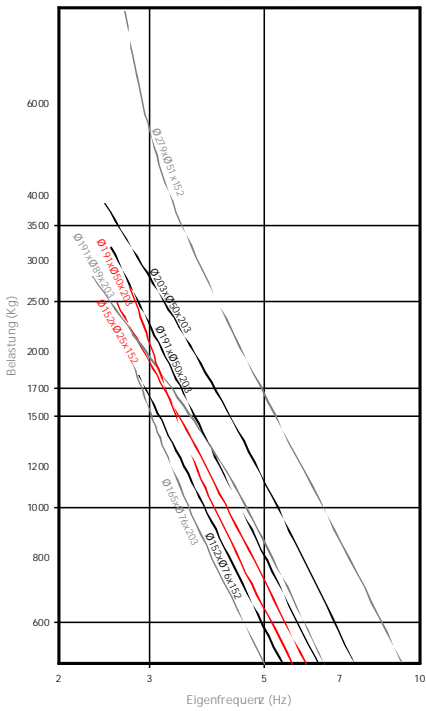
EIGENFREQUENZEN AMC MECANOCAUCHO® VERSTÄRKTE ELASTOMERFEDERN Ø152 - Ø279
